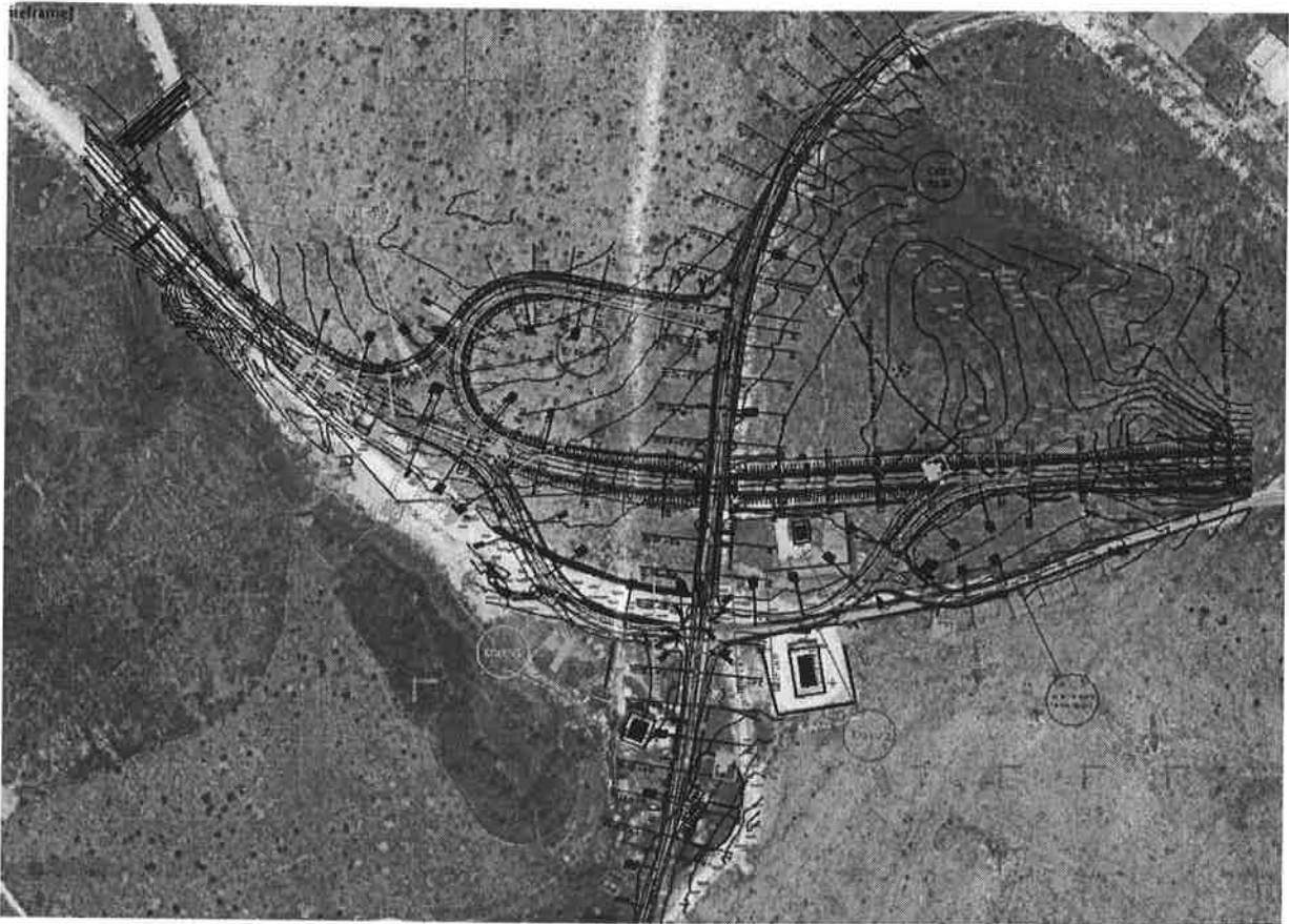
Slika 1: Situaciono rješenje Raskrižja Varda (Glavni projekat Južne obilaznice Mostara, 2015)
